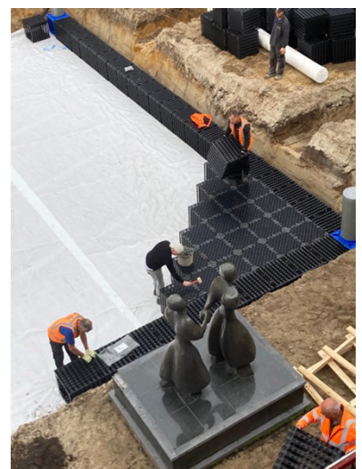
Afbeelding: kratten infiltratiesysteem Raadhuisplaza
